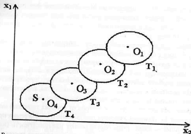
Рис. 3.1. Возрастные изменения в положениях аттракторов для их центров O_1 - O_4 при переходе от возраста T_1 (юность) к возрасту T_4 (старость). Здесь координаты x_1 и x_2 - любые параметры физического состояния фазотона мозга человека на севере РФ.
