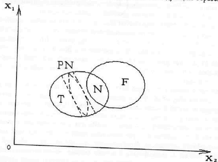
Рис. 2.1. Фазовый портрет изменения уровня сухожильного рефлекса ( x_1 ) от уровня катехоламинов ( x_2 ), где F – физическая патология, T – тоническая патология, N – норма, PN – псевдонорма.
